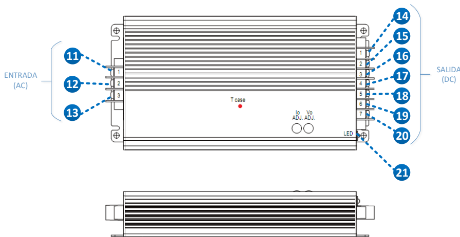
Fig. 4 Cargador de baterías/ Battery charger.
