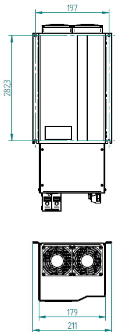
Dimensiones EPCL 5K5
