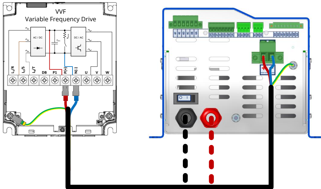
Fig. 28 Conexión entre Convertidor DC/DC y variador de velocidad/ DC/DC converter to VVVF Drive connection.
